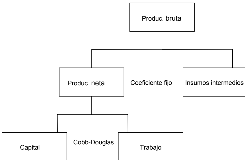
Gráfica 1: Estructura anidada de las Funciones de Producción
